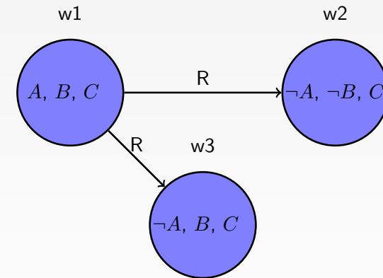
A, B, C, \dots aussagenlogische Variablen; blaue Kugel: Interpretation
